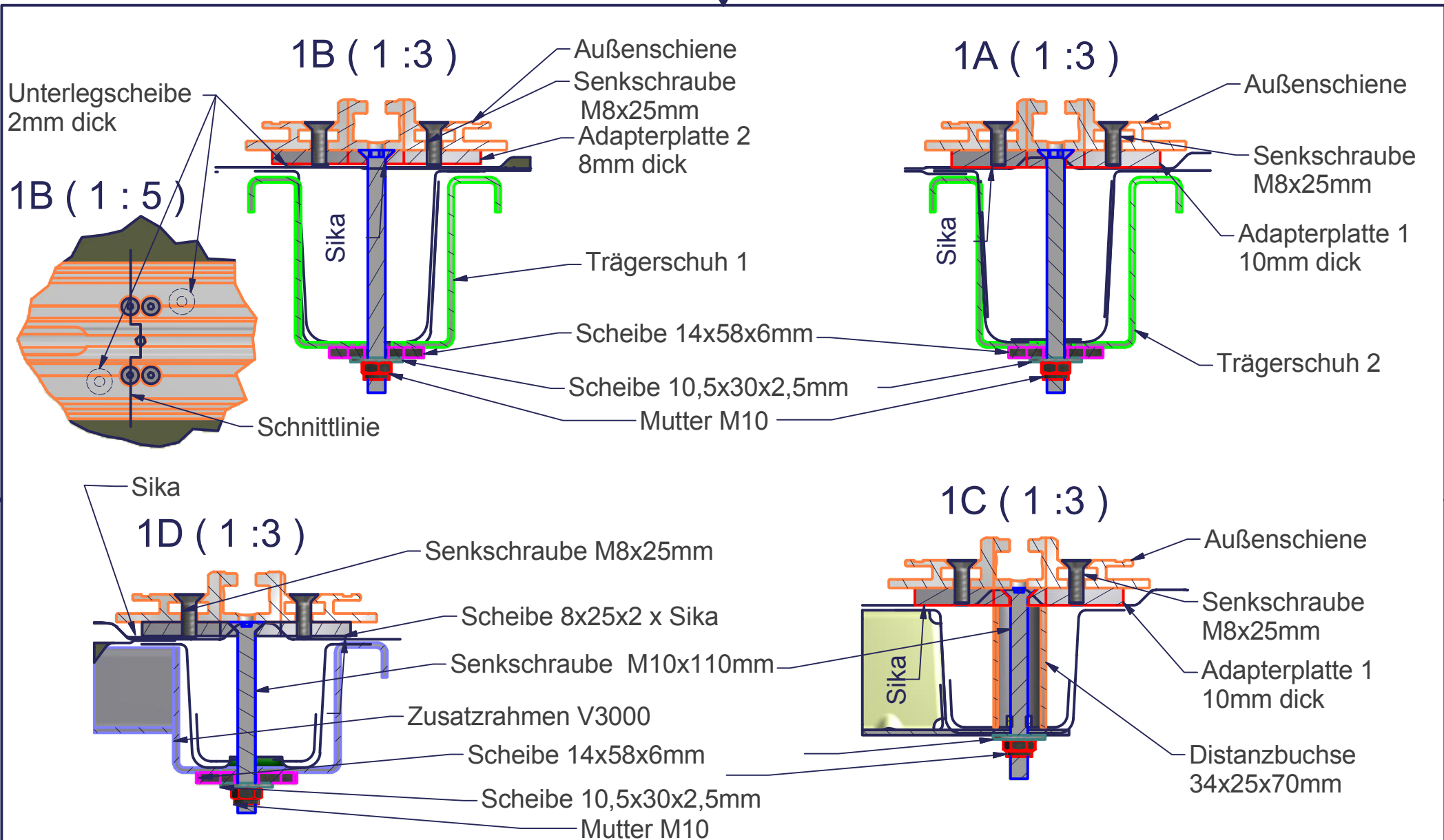
Schnitte Befestigung Außenschiene
