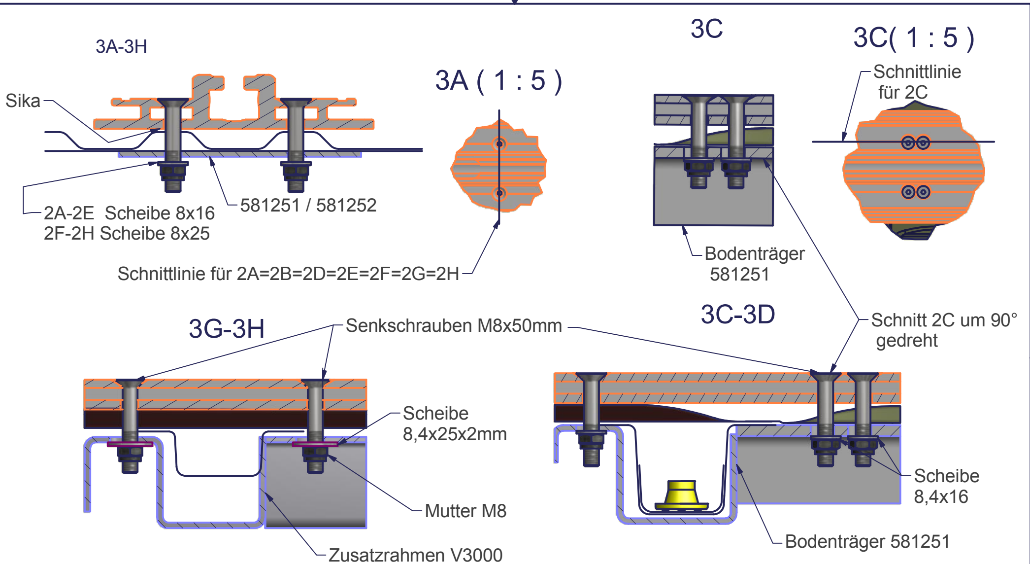
Schnitte Befestigung Innenschiene
